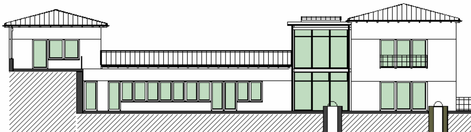
Ansicht Süd
